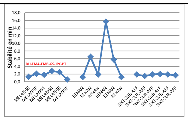
Figure 8 : Stabilité de la résistance de la pâte au pétrissage au Farinographe
