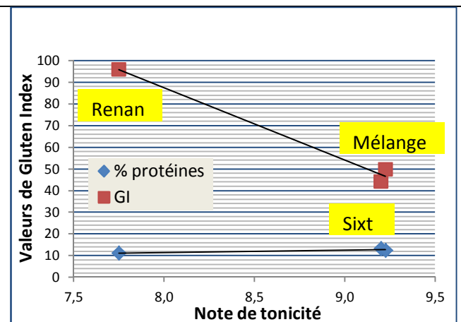
Figure 16 : Relations Gluten Index-protéines et tonicité au façonnage
