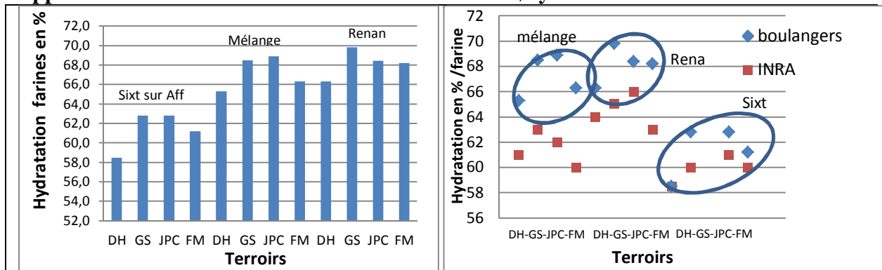
Figure 9 : Hydratation des farines par les expérimentateurs boulangers
